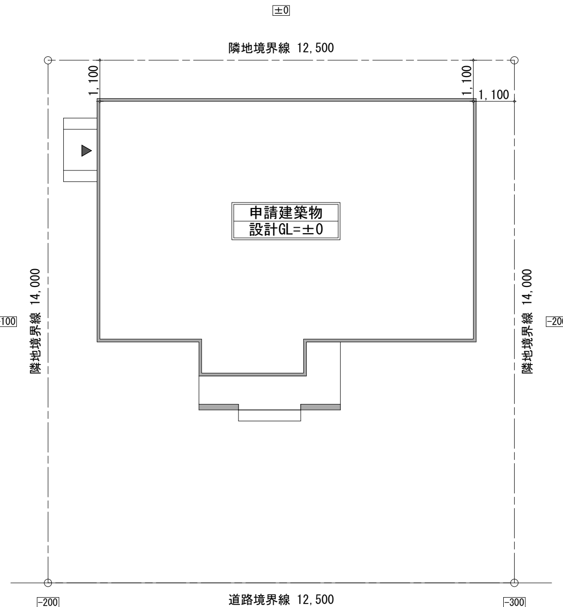
建物配置図 S=1/100
